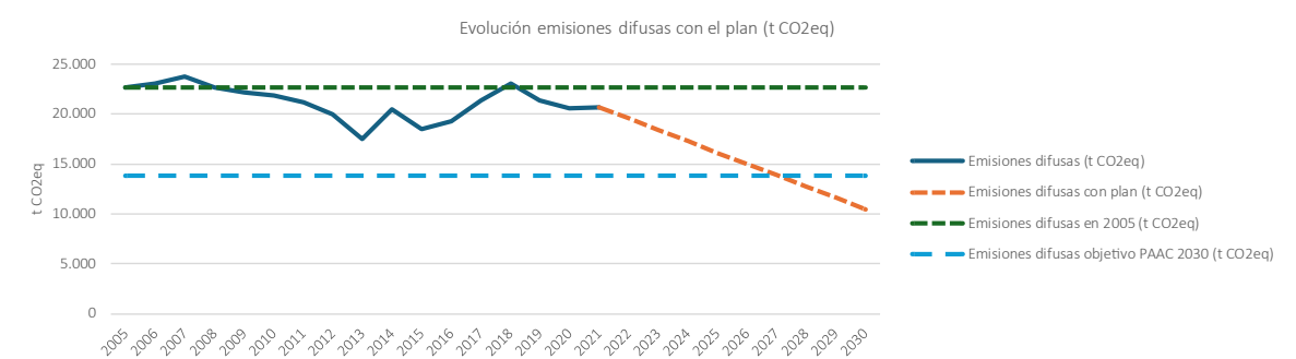
Figura 61. Evolución de emisiones difusas esperadas en La Roda de Andalucía con la aplicación del PMCC.
