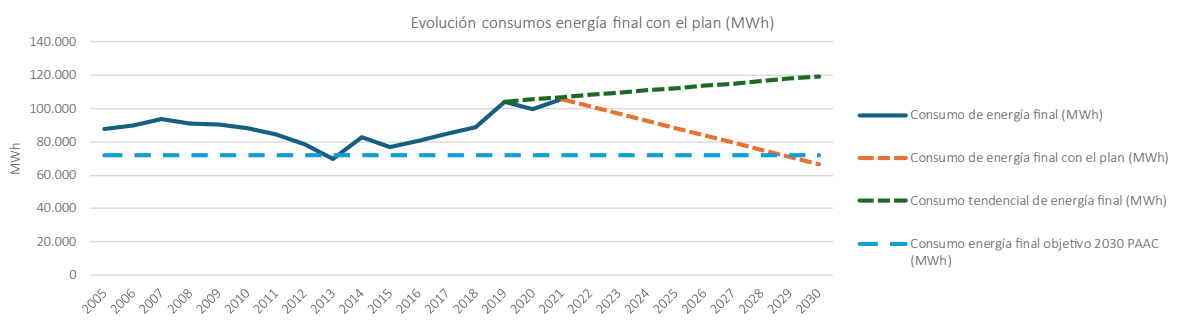
Figura 62. Evolución de los consumos de energía final esperadas en La Roda de Andalucía con la aplicación del PMCC.
