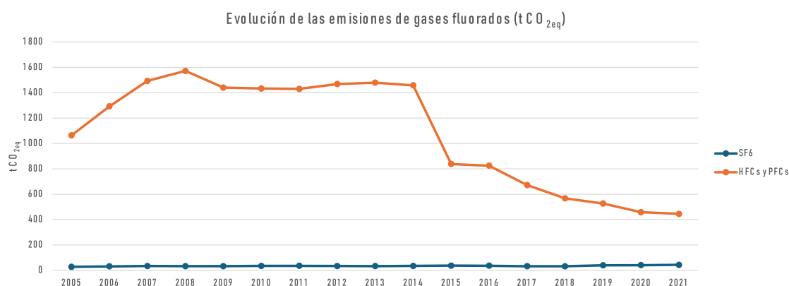
Figura 17. Evolución de las emisiones de los gases fluorados por tipo de 2005 a 2021.
