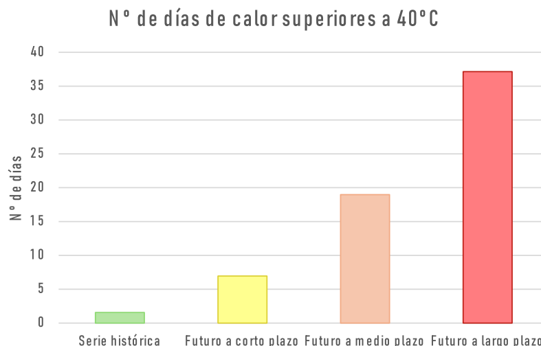
Figura 39. Diagrama de variación del número de días en los que se superan los 40 °C al año en La Roda de Andalucía para la serie histórica de 1961 a 1990 y para los horizontes temporales de futuro a corto, medio y largo plazo. Fuente: Elaboración propia a partir de datos del Visor de escenarios climáticos en Andalucía (2024)
